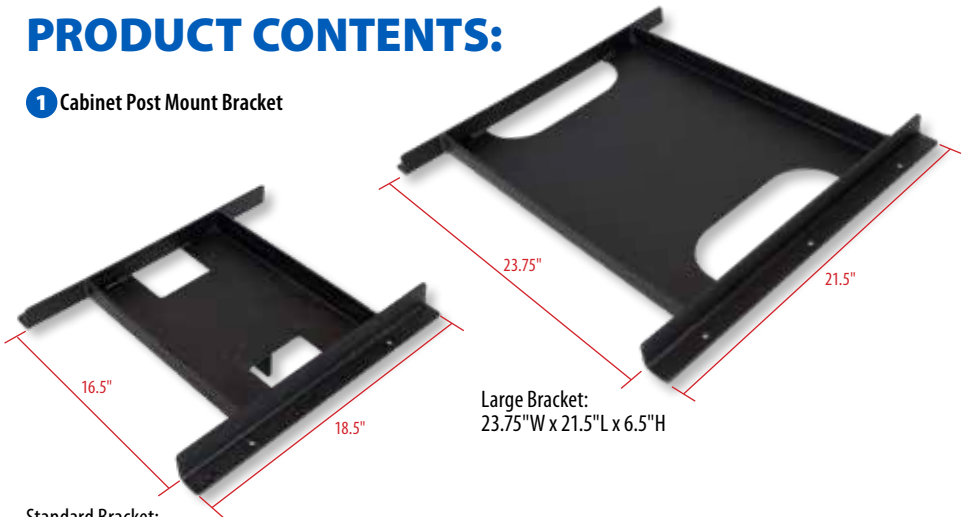
Standard Bracket: 16.5"W x 18.5"L x 6.5"H
